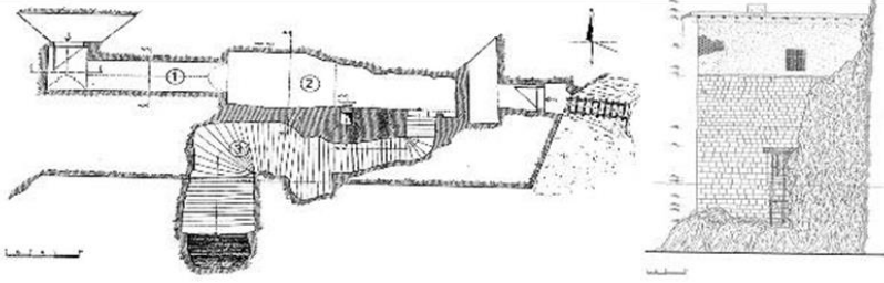
Şekil 5,6. Sarnıç Planı ve Doğu Cephesi (Ş. Öztürk)
