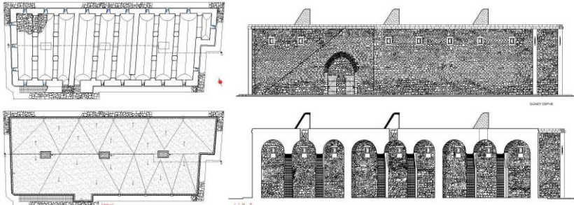
Şekil 69-72. Miri Ambarı Plan-Örtü Sistemi-Kesit ve Güney Cephesi (Ş. Öztürk)
