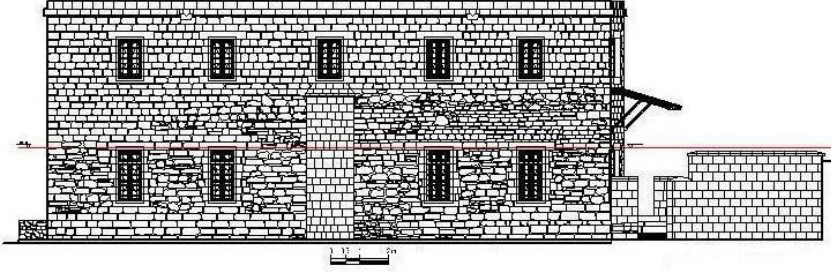
Şekil 92. Horhor Cami Güney Cephesi (Ş. Öztürk)
