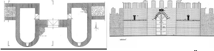
Şekil 24,25. Saray Kapı Plan ve Güney Cephesi (Ş. Öztürk)
