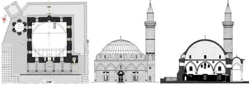
Şekil 37-39. Hüsrev Paşa Camii Planı, Kuzey Cephe ve Kesiti (Ş. Öztürk)
