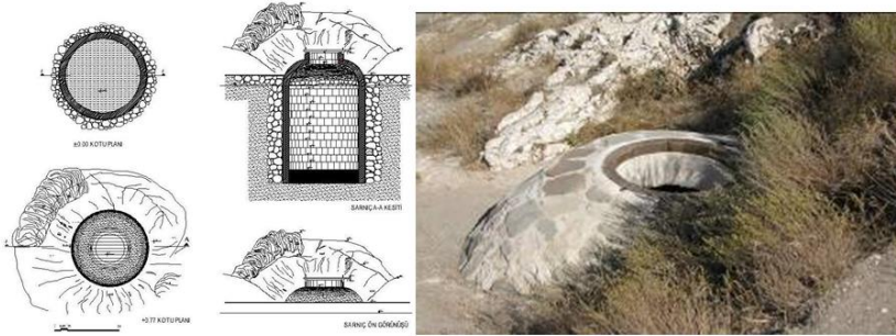
Şekil 15-17. Kale Üstü Sarnıcı Planı-Kesit ve Genel Görünüşü (Ş. Öztürk)
