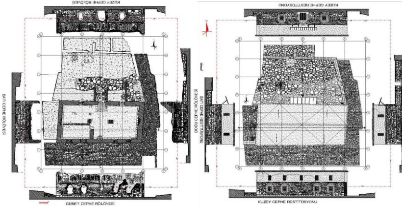
Şekil 93,94. Abbasağa Camii Rölöve ve Restitüsyon Vaziyet Planı (Ş. Öztürk)
