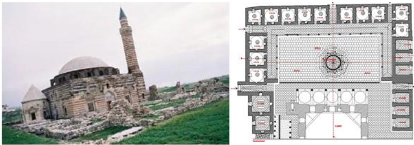
Şekil 43,44. Hüsrev Paşa Medrese Kuzeydoğu Görünüşü ve Planı (Ş. Öztürk)
