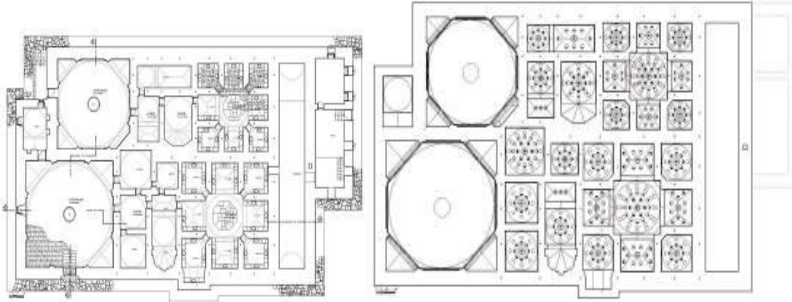
Şekil 54, 55. Hüseyin Paşa Külliyesi Çifte Hamamı Planları (Ş. Öztürk)
