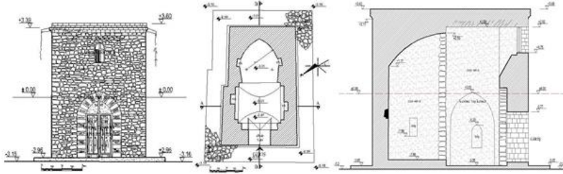
Şekil 77-79. Surp Diziranavor Kilisesi (Şapel) Plan, Kesit ve Batı Cehesi (Ş. Öztürk)
