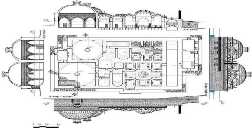
Şekil 53. Hüsrev Paşa Külliyesi Çifte Hamam Planı, Kesit ve Cepheleri (Ş. Öztürk)
