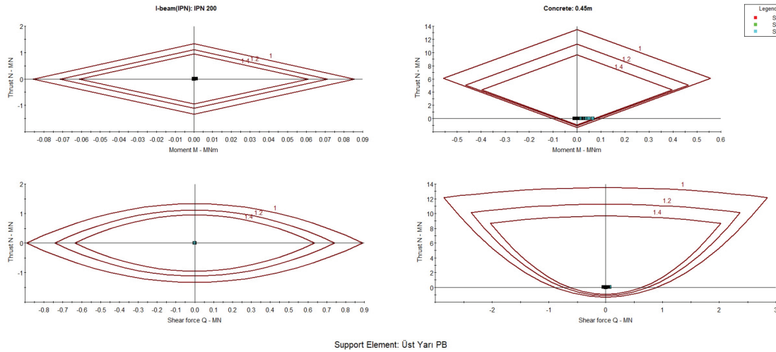
Şekil 28. Tarama kazısı sonrası tahkimat kapasite eğrileri.
