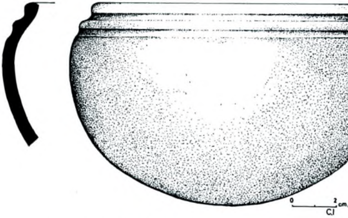
Çiz. 8— Urne kapağı olarak kullanılan çanak. 1 no'lu gömüt Zeich. 8— Schale; sie diente als Urnendeckel, Grab 1
