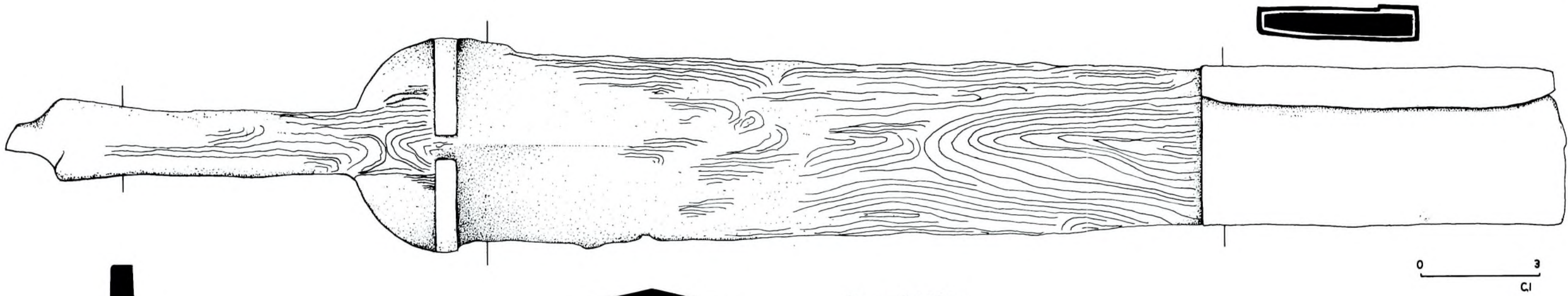
Çiz. 12 — Dedeli Kılıcı Zeich. 12 — Dolch von Dedeli
