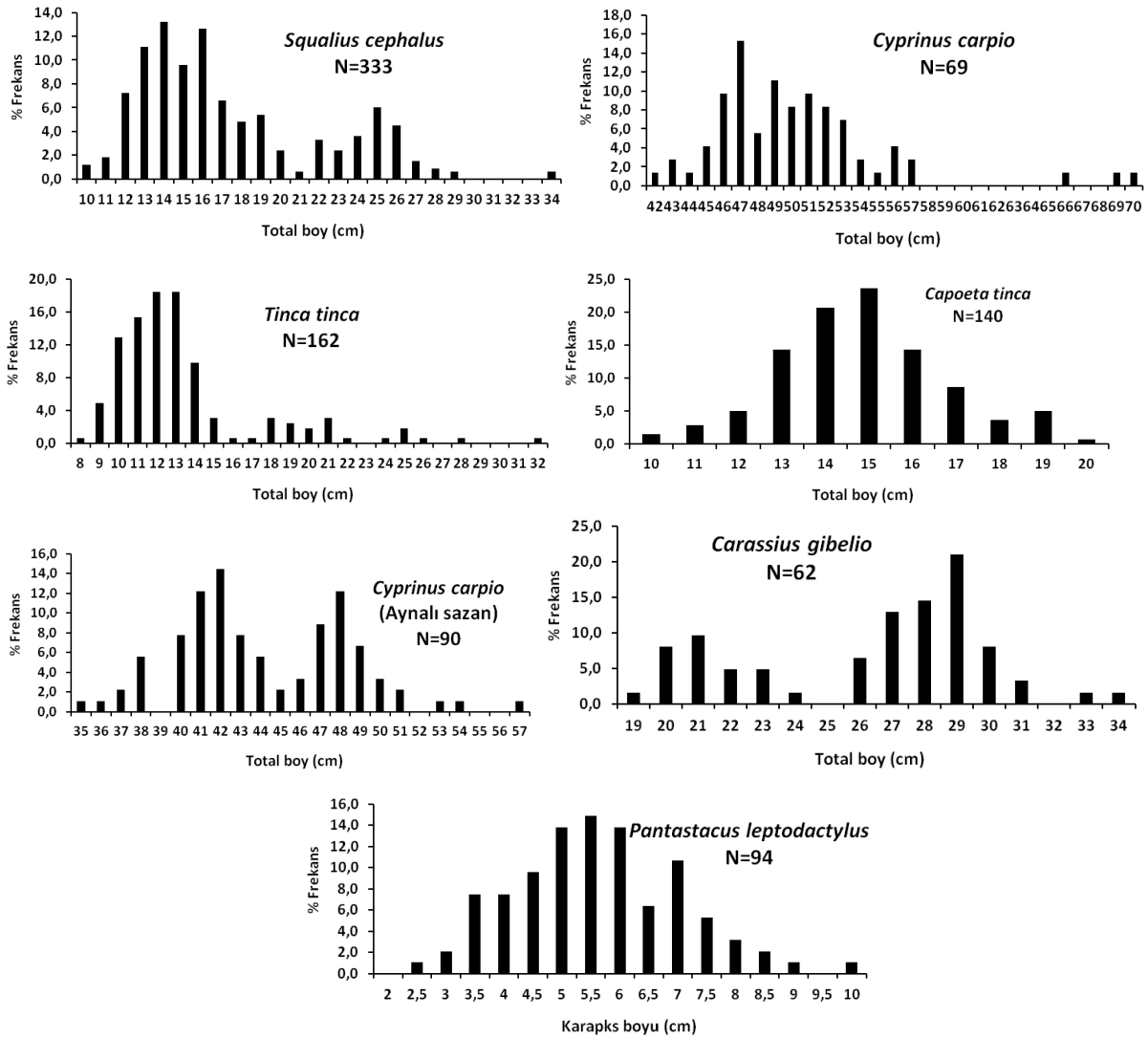
Şekil 3. Yeniçağa gölündeki makrofaunanın boy-frekans dağılımları
