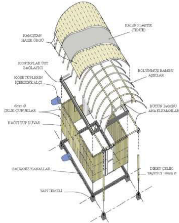
Şekil 15. Alçı Dolgulu Kağıt Tüplerden Barınak Örneği Sistem Perspektifi (Usl 15).
