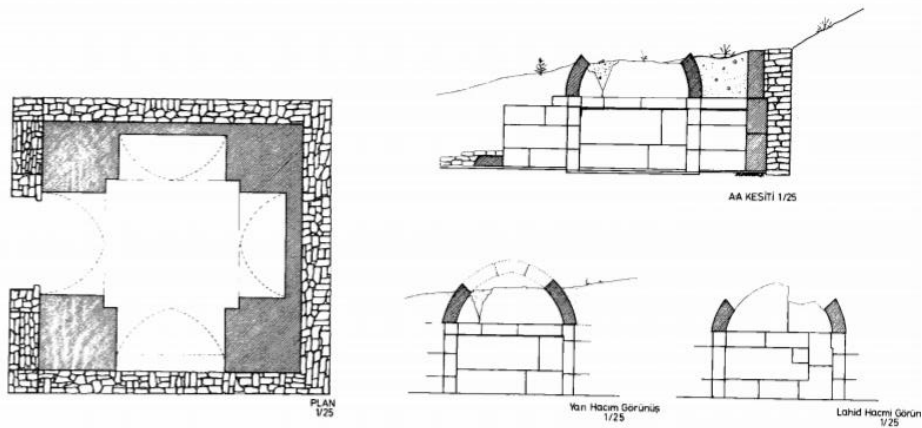
Resim 5: Aizanoi Güney Nekropolis Nişli Mezar Çizimi (Türktüzün 1992, 86, Çizim 1)
