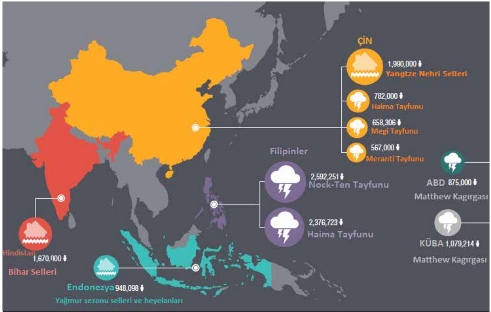
Şekil 4:2016'da İklim Değişikliği Sebebiyle Gerçekleşen En Büyük 10 Yer Değiştirme, Kaynak: (Stapleton, Nadin, Watson, & Kellett, 2017: 10)
