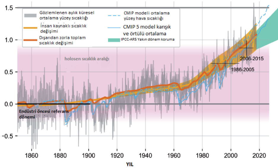
Şekil 2: 1850-1900'e Göre Sıcaklık Değişimi. Kaynak: IPCC 1,5°C Küresel Isınma Özel Raporu (IPCC, 2018)¹
