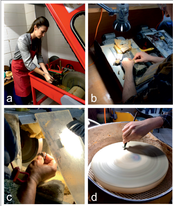
Şekil 6. a) Büyük dilimleme, b) Küçük dilimleme, c) Taşlama işlemi, d) Cila işlemi.
