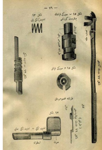
(Şekil 12) Emniyet Tetiği-Emniyet Tetiği Sapı (Şekil 12 B) Emniyet Tetiği (Şekil 13) Emniyet Tetiği Yay (Şekil 15 B) Sürgü kapağının yukarıdan görünüşü-Kuyruk Tırnağa Mahsus Yatak (Şekil 15 H) Sürgü Kapağı Tırnağa Mahsus Yatak (Şekil 16) (tırnak) Fişenk Çıkaracağı Dış (Şekil 17) Fişenk Atacağı ..... Halka Kanal
