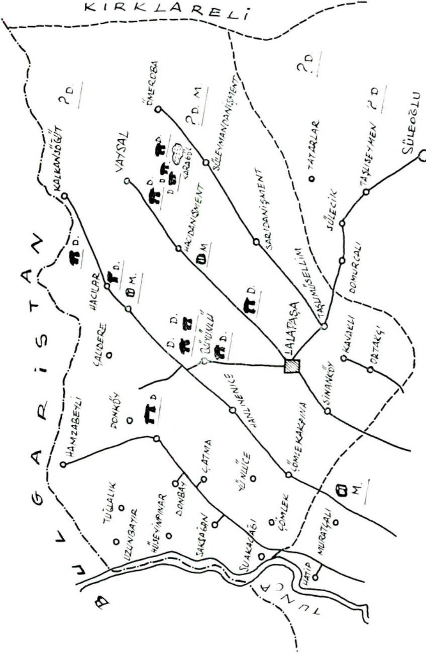
Lalapaşa (Edirne) yöresindeki Dolmen ve dikilitaşların dağılışı, (Ruhi Esmi'ne göre).
