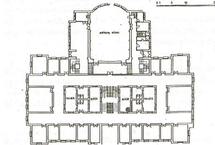
Şekil 7. Eski Adliye Sarayı Zemin Kat Planı (Aslanoğlu, 2001: 138)
