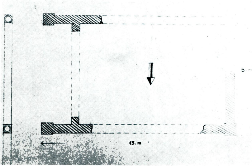
Res. 25 — Büyük mabed, Prostilos tipinde
