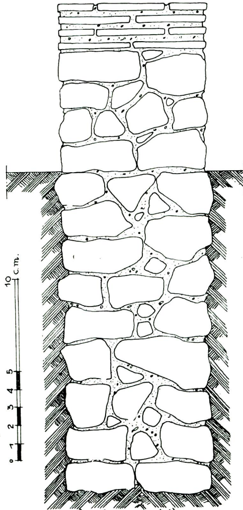
Bir duvar kesiti
