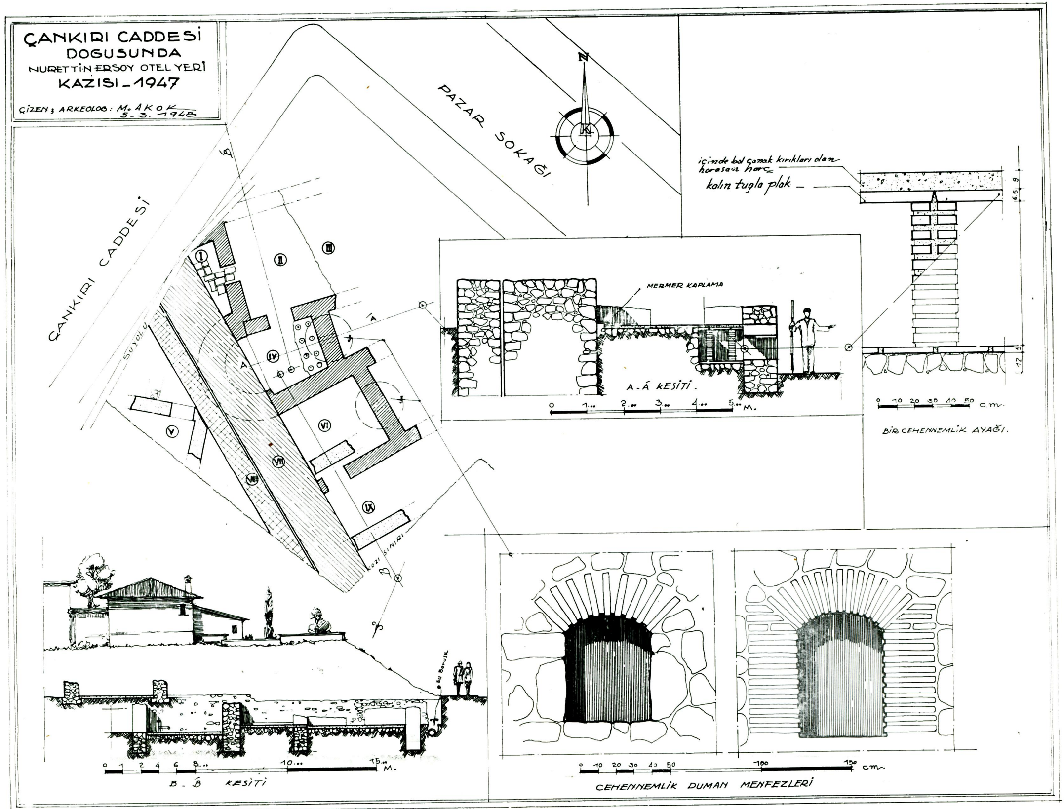
Res. 7 — Çankırı Caddesi doğusundaki buluntu yerinde görülen mimarlığın genel plânı.
