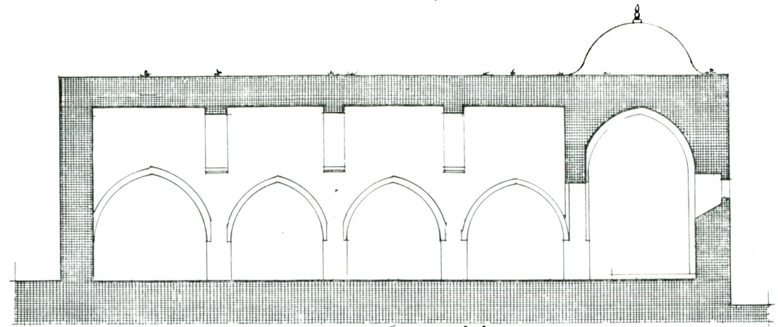
C, C KESİTİ
