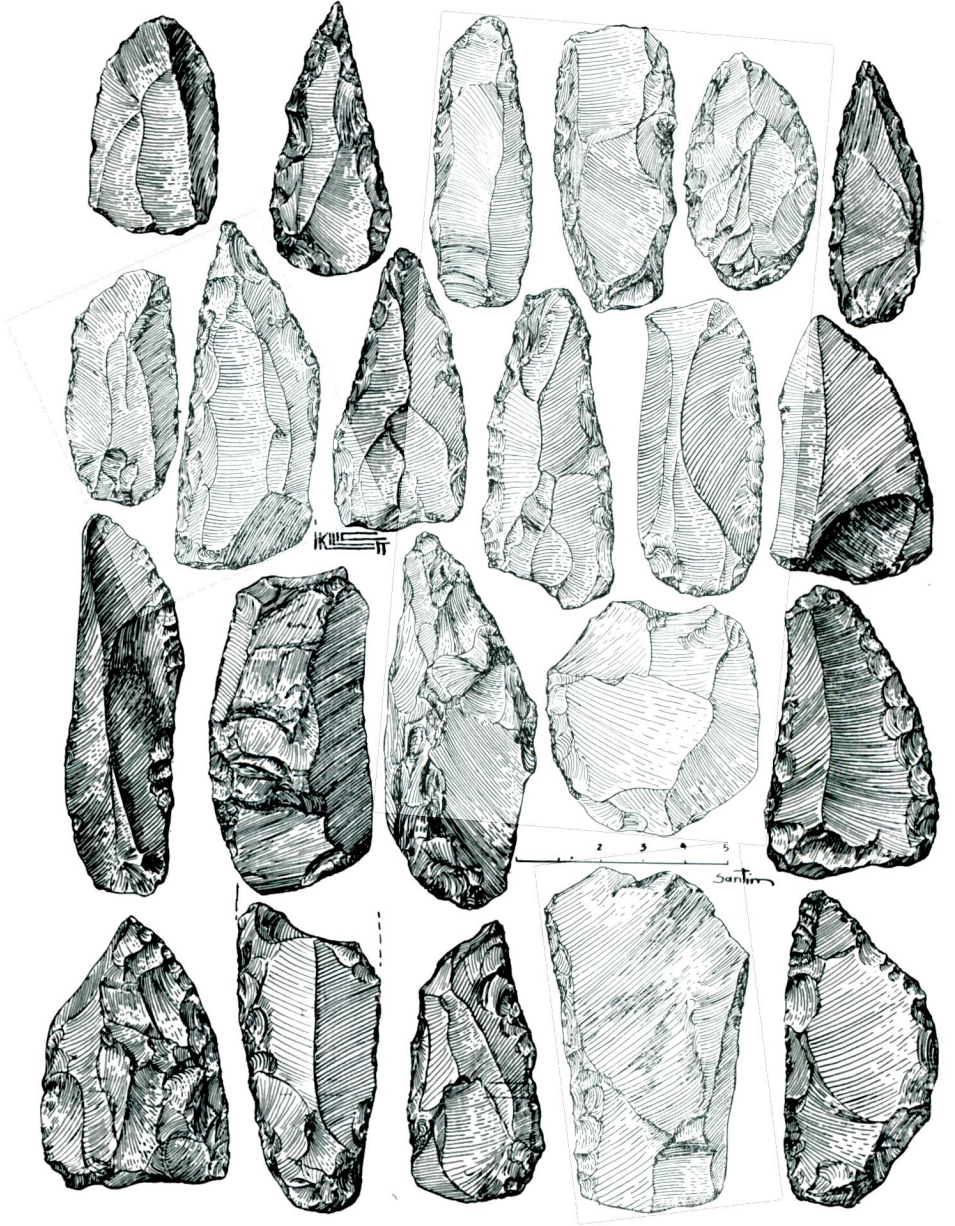
Karain Mağarası 1954 yılı hafriyat çukurundan Orta Paleolitik. Musteriye II sileks aletlerinden birkaç örnek.
