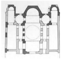
Şekil 13. Restitüsyon planı (Ousterhout ve Bakirtzis, 2007)
