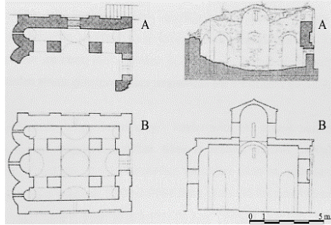
Şekil 72. Planı ve kesiti (A: Rölöve, B: Restitüsyon) (Mamalukos, 2004; Sarıoğlu, 2021)
