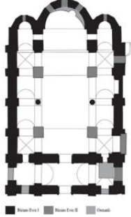
Şekil 53. Zemin kat planı (Bauer ve Klein, 2006)
