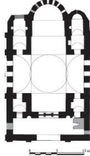
Şekil 54. Üst kat planı (Bauer ve Klein, 2006)
