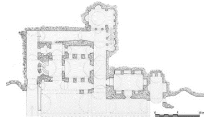
Şekil 77. Planı (Eyice, 1969)
