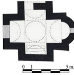
Şekil 23. Planı (Eyice, 1969)
