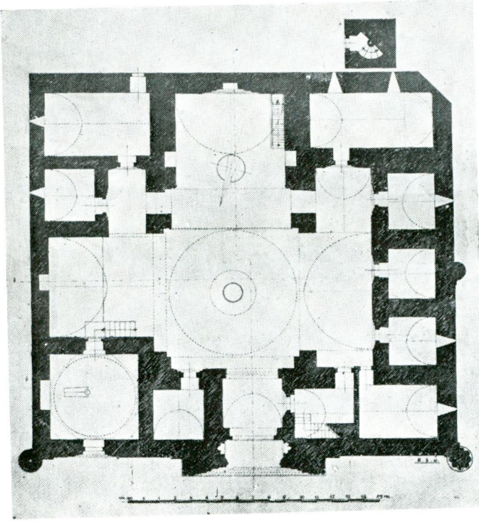
Res. 1 — Cacadbey Medresesi'nin genel plânı. (Bk. A. Saim Ülgen, Vakıflar Dergisi, sayı 2, s. 261, Res. 1).
