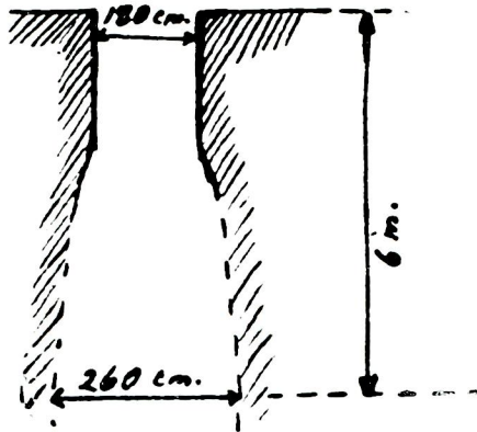
Res. 2 — Kuyu çapının aşağı doğru genişlemesi.
