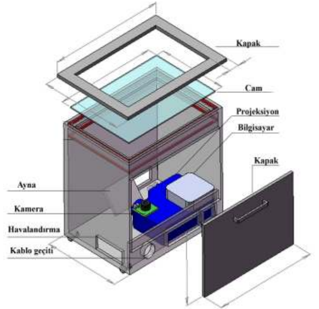
Şekil 5. Sistem düzeneği
