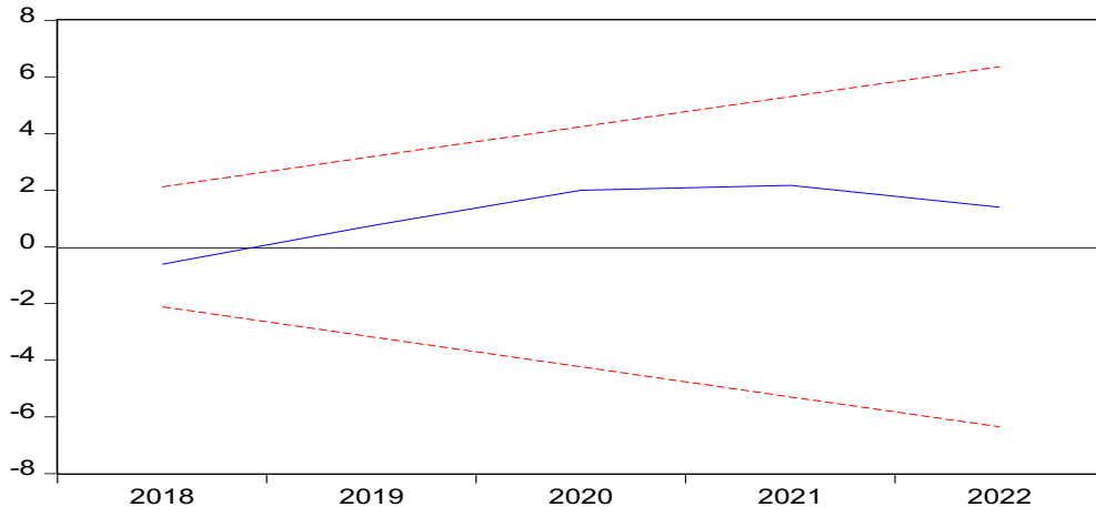
Şekil 4. CUSUM Testi
