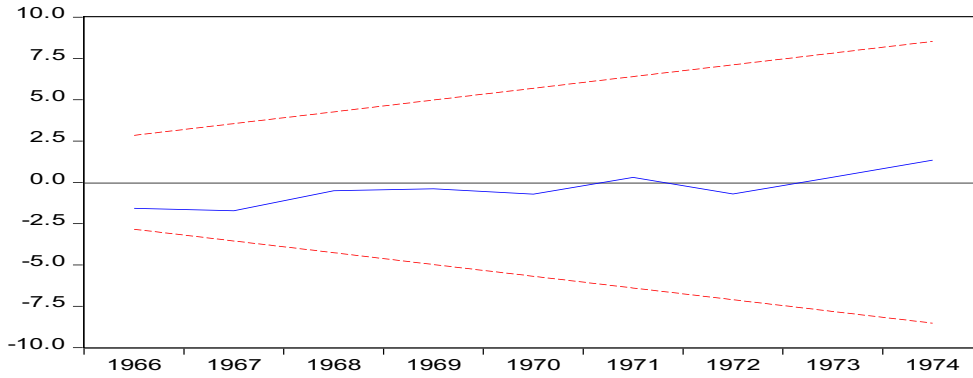
Şekil 1. CUSUM Testi
