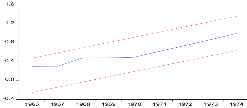
Şekil 2. CUSUMSQ Testi
