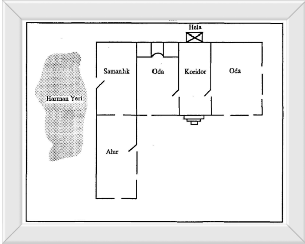
Şekil 4. Merzifon İlçesinde Yamaç ve Dağ Meskenleri Yaygın Tek Katlı Ev Planı (ölçeksiz)
