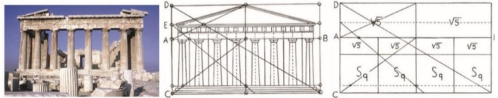
Şekil 1. Parthenon cephesine yönelik yapılan altın oran uyum çalışması (Ghyka, 1977)
