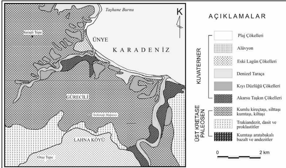
Şekil 2. Çalışma alanı ve çevresinin jeoloji haritası
