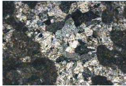
Şekil 8. Örnekte yeralan erime boşlukları tamamen kalsit çimento ile doldurulmuş olup (açık renkli alanlar) kayada gözeneklilik bulunmamaktadır (Büyütme: 10x).
