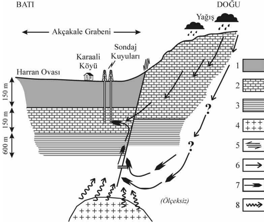
Şekil 4. Karaali Köyü civarı şematik jeoloji kesiti [1- Adıyaman Formasyonu (Pliosen, kil, marn, kum ve çakıl ardalanması, örtü kayaç), 2- Fırat Formasyonu (Üst Eosen-Alt Miyosen, kırıklı-çatlaklı ve erime boşluklu kireçtaşı, rezervuar kayaç), 3- Gaziantep Formasyonu (Alt Eosen, çörtlü, killi kireçtaşı, marn ardalanması), 4- Magmatik sokulum (ısı kaynağı), 5- Fay, 6- Soğuksu sirkülasyonu, 7- Sıcaksu sirkülasyonu, 8- Isı taşınımı].
