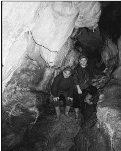
Şekil 9. Yazkonağı Mağarası'nın ikinci galerisindeki sarkıt ve diktler
