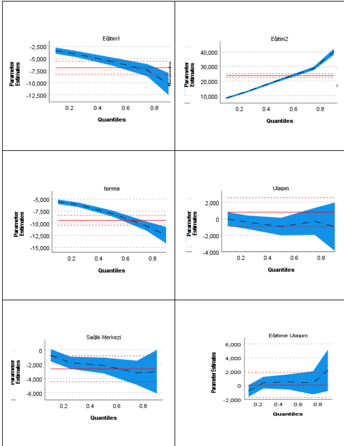
Şekil 1. Kantil Regresyon Tahminlerinin Grafikleri
