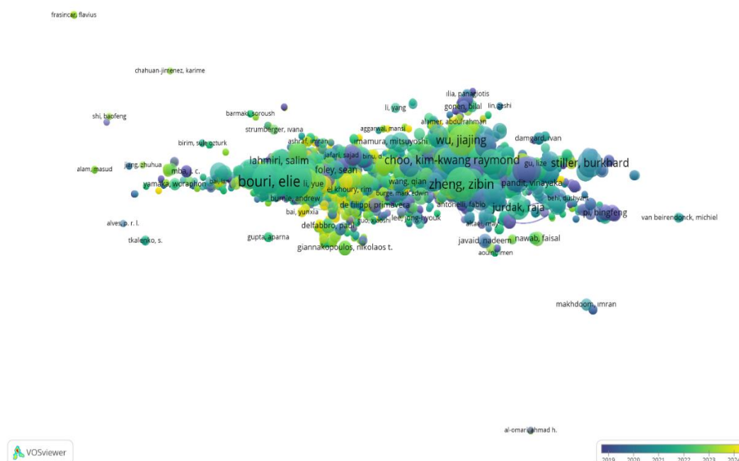
Şekil 2. Yazar atıf analizi yoğunluk analizi
