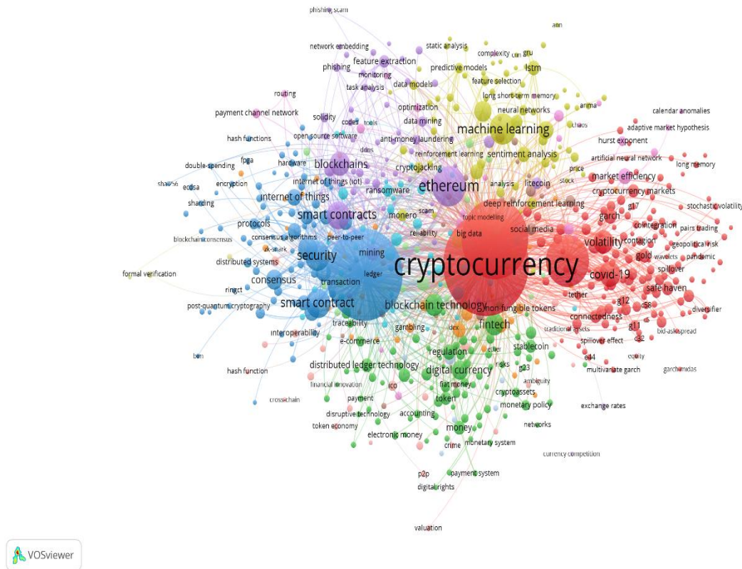
Şekil 7. Anahtar kelime analizi
