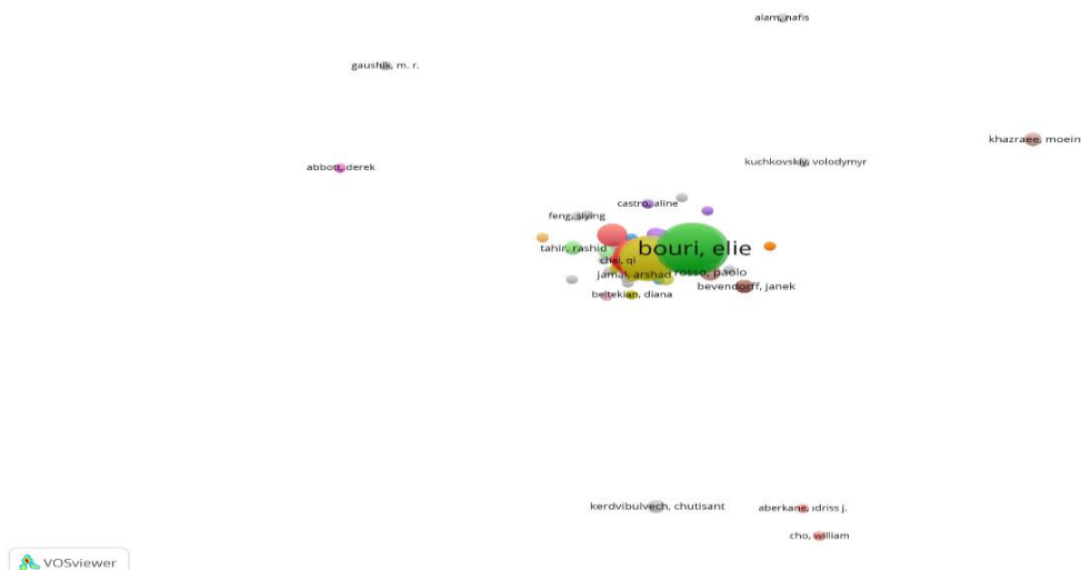
Şekil 8: Bibliyografik eşleşme analizi
