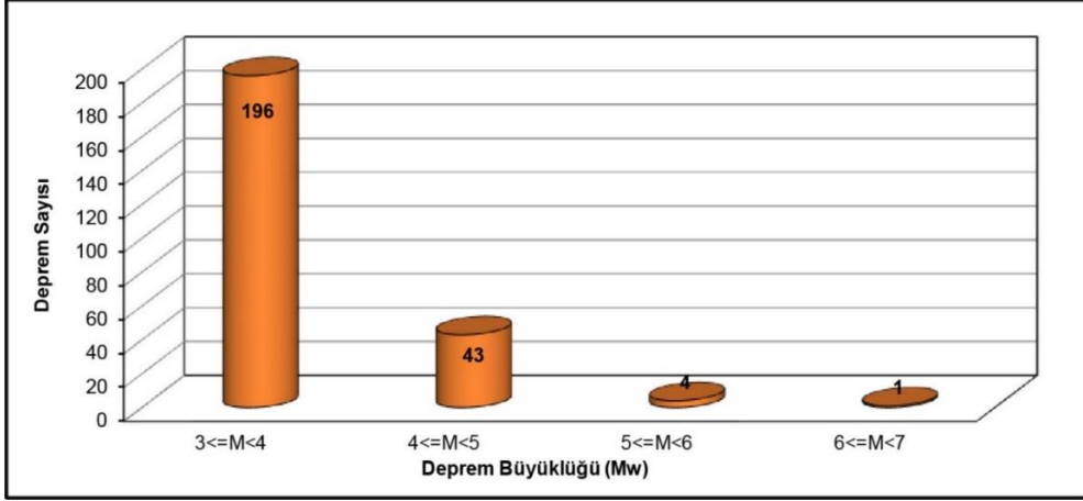
Şekil 1. 24 Ocak 2020 Sivrice-Elazığ depremi ve sonrasında oluşan depremlerin ( m \geq 3 ) sayı-magnitüd ilişkileri (Deprem verileri Kandilli Rasathanesi ve Deprem Araştırma Enstitüsü'ne ait olup 19.06.2020 saat 14:38'e kadar oluşan depremleri ( m \geq 3 ) kapsamaktadır)
