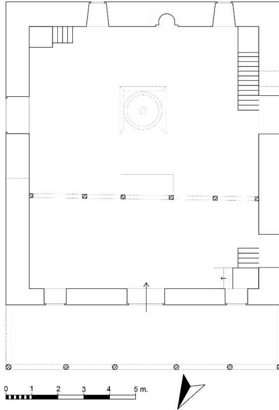
Plân 1: Yassihöyük Camisi Plâni (M. Canseven)
